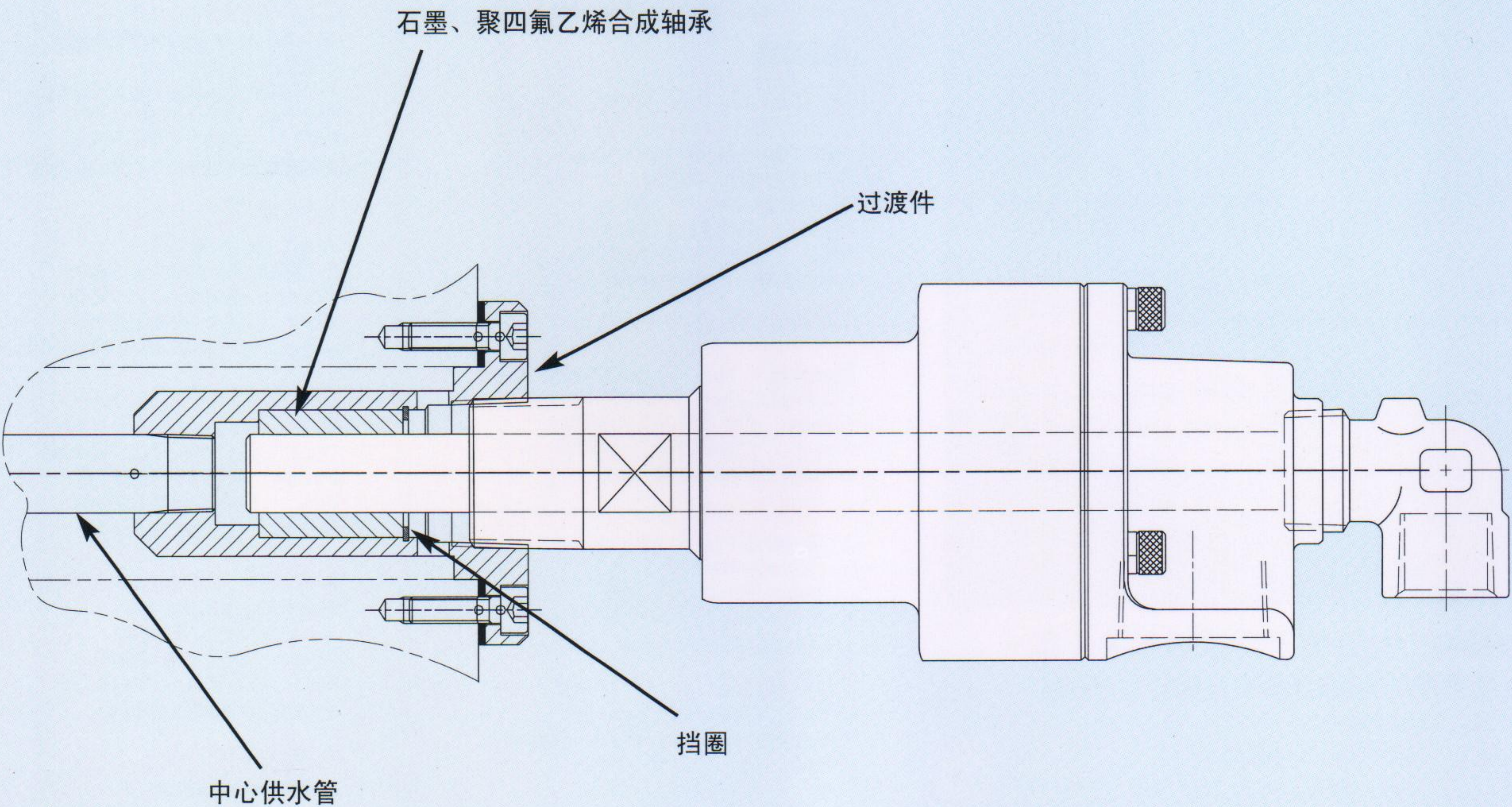
外部安装示意图
